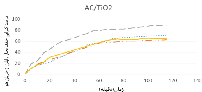
شکل ۲: کارایی حذف زایلین در نسبت‌های مختلف از AC/TiO 2
