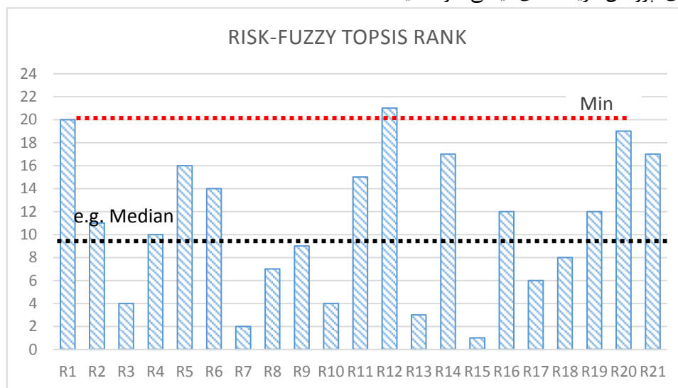
نمودار ۲. نمودار رتبه ریسک‌های ایمنی در پروژه‌های ساختمانی محاسبه شده با روش TOPSIS فاز۱
