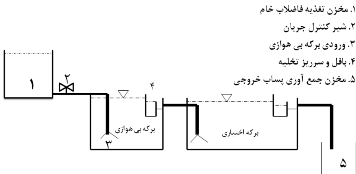
شکل ۱- شماتیک سیستم برکه ای
