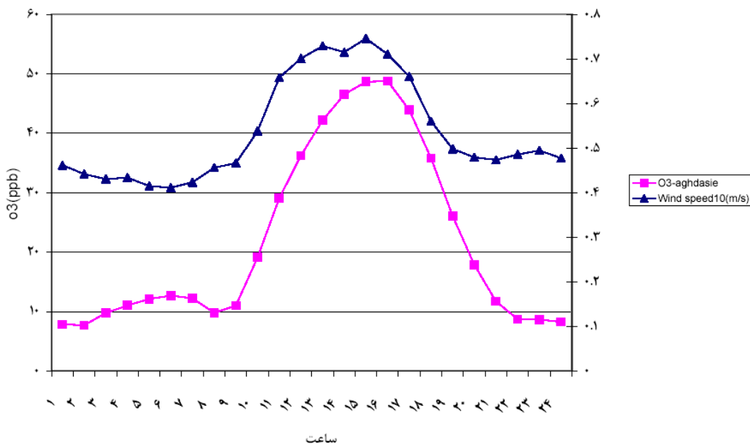
نمودار ۴- تغییرات میانگین ساعتی غلظت ازن با تغییرات میانگین ساعتی سرعت باد در ایستگاه اقدسیه
