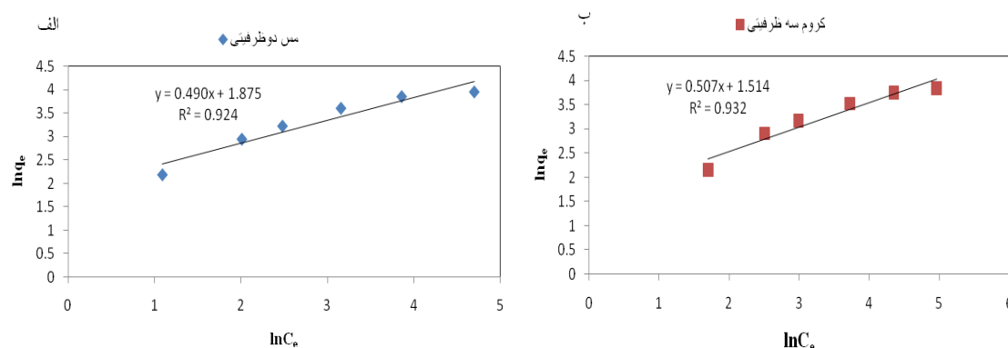
نمودار ۶- جذب سطحی فلزات (الف) مس دو ظرفیتی و (ب) کروم سه ظرفیتی
