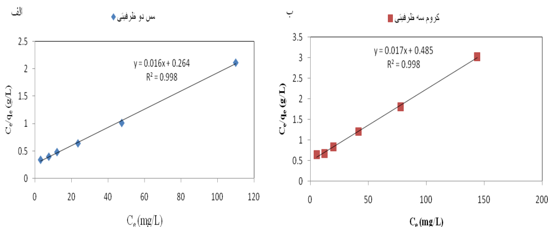
نمودار ۵- جذب سطحی فلزات (الف) مس دو ظرفیتی و (ب) کروم سه ظرفیتی توسط سبوس برنج بر اساس مدل لانگمویر
