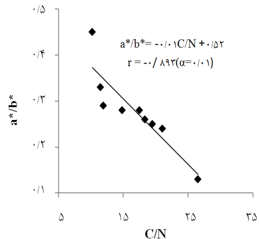
شکل ۵- ارتباط میان نسبت C/N و پارامتر a^*/b^*
