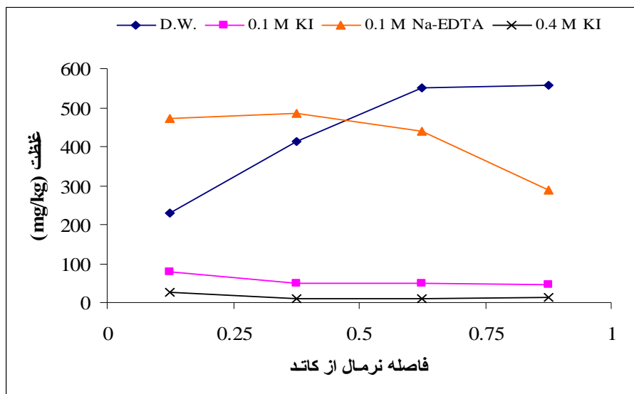
شکل (۵) غلظت جیوه موجود در خاک آلوده مصنوعی با گرادیان ولتاژ ۱/۵ VDC/cm
