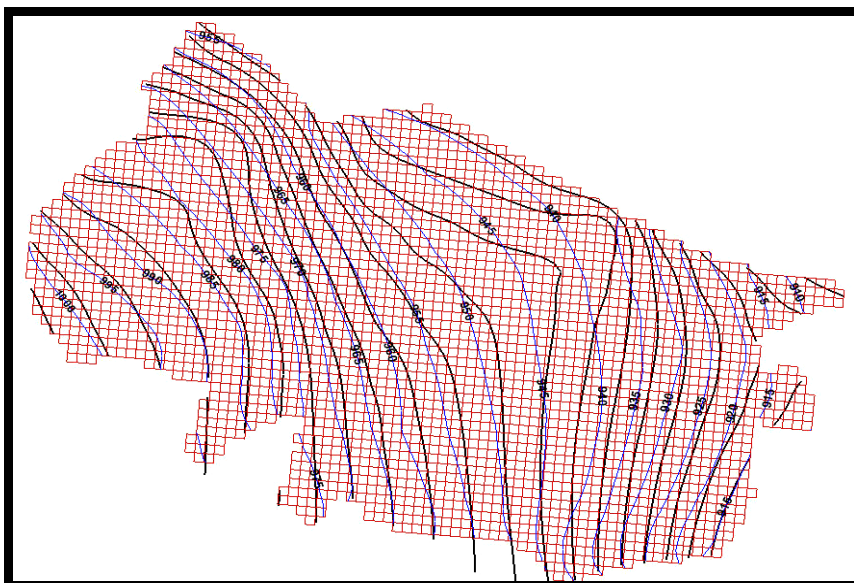
نقشه ۶- منحنی های هم پتانسیل شبیه سازی شده (آبی) و منحنی های اولیه سطح آب زیرزمینی (مشکی) ( گام زمانی دوازدهم - دوره تنش دوم)
