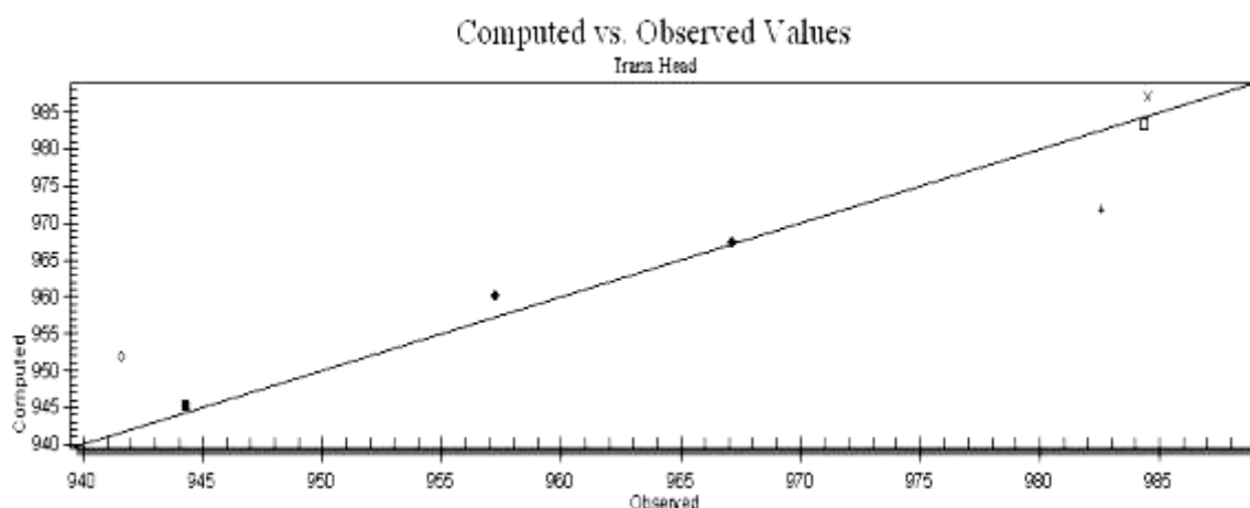
شکل ۵- اسکاتر دیاگرام سطح آب مشاهده شده و شبیه سازی شده در محل چاه های مشاهده ای آبخوان شهری مشهد ( گام زمانی دوازدهم - دوره تنش دوم)
