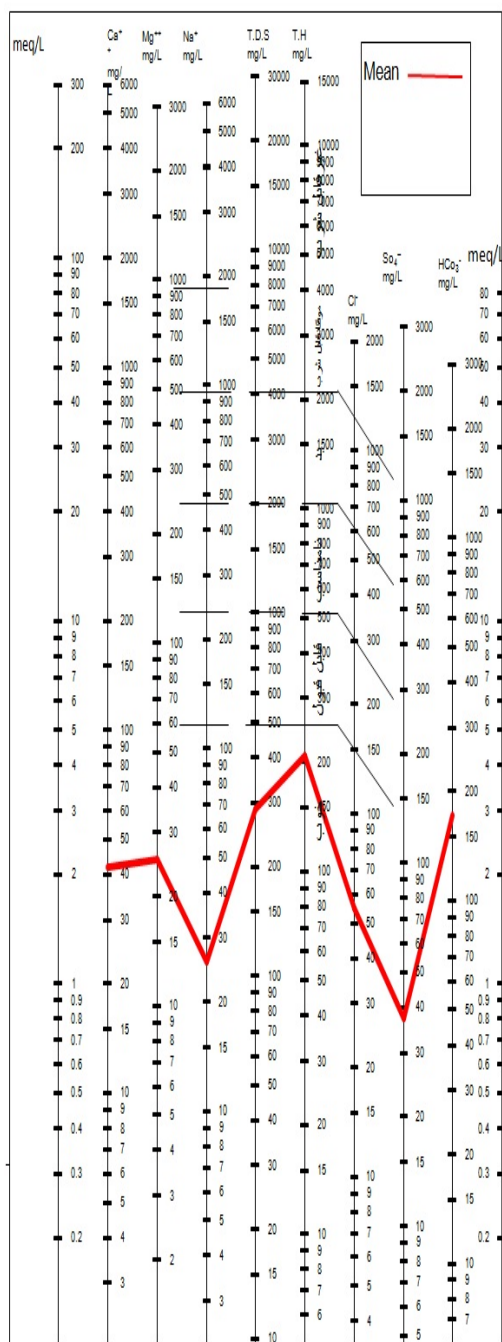
نمودار ۱۰- دیاگرام شولبر برای چاه آب شرب منطقه ی انباج (آذر)
