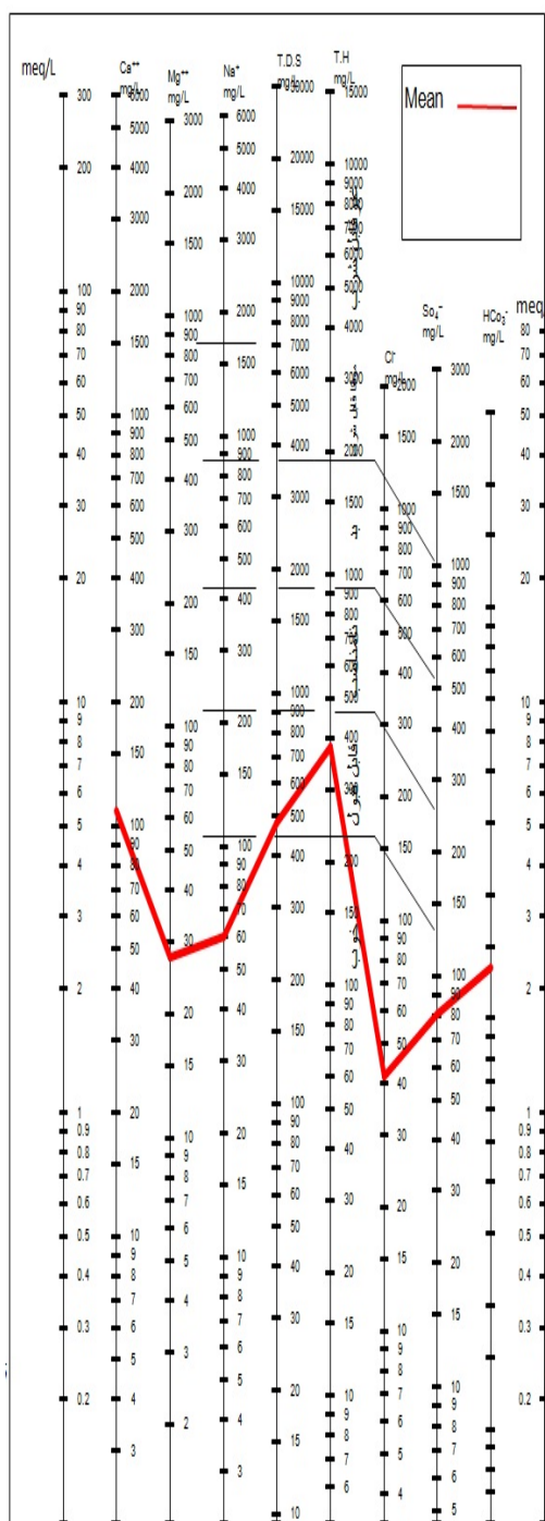
نمودار ۱۱- دیاگرام شولر برای چاه آب شرب منطقه ی
