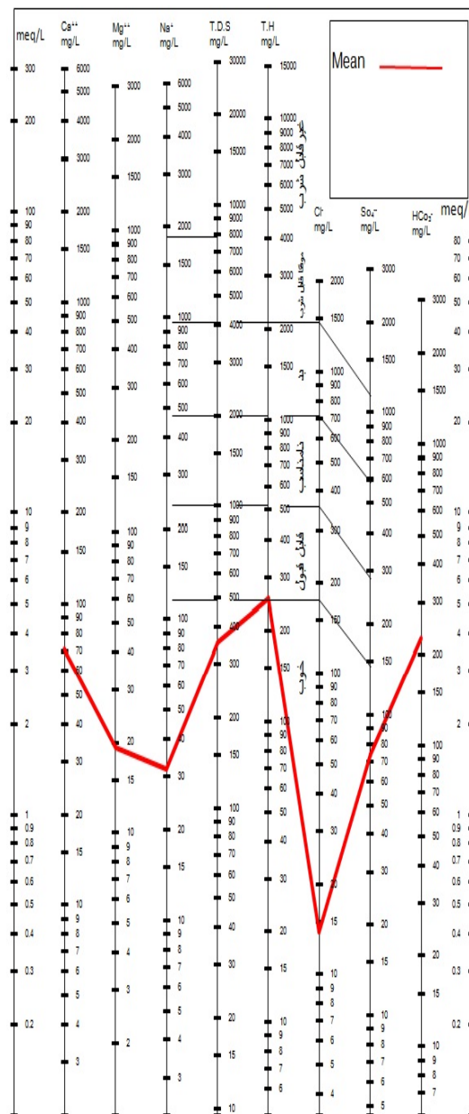
نمودار ۷- دیاگرام شولبرای چاه آب شرب منطقه ی هنزک
