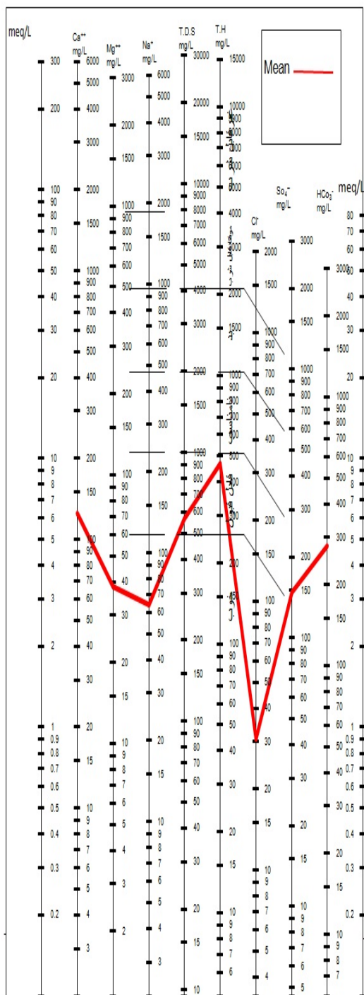
نمودار ۱۴- دیاگرام شولبر برای چاه آب شرب منطقه ی کند سفلا (آذر)
