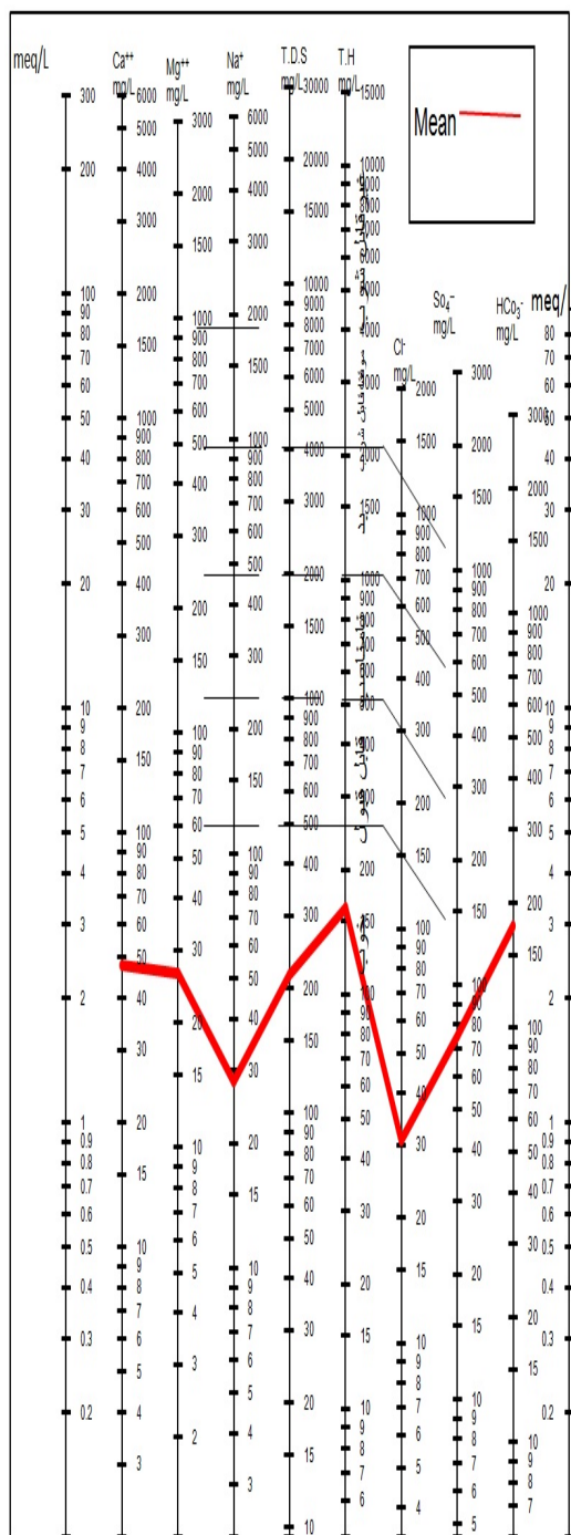
نمودار ۱۲- دیاگرام شولر برای چاه آب شرب منطقه ی
