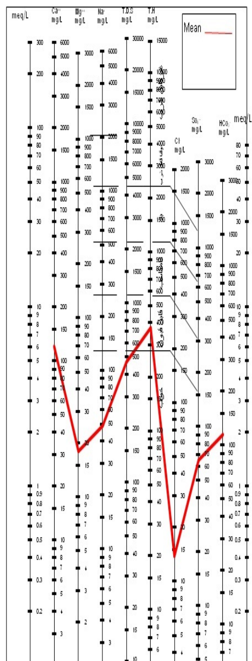
نمودار ۹- دیاگرام شولبر برای چاه آب شرب منطقه ی انباج (تیر)
