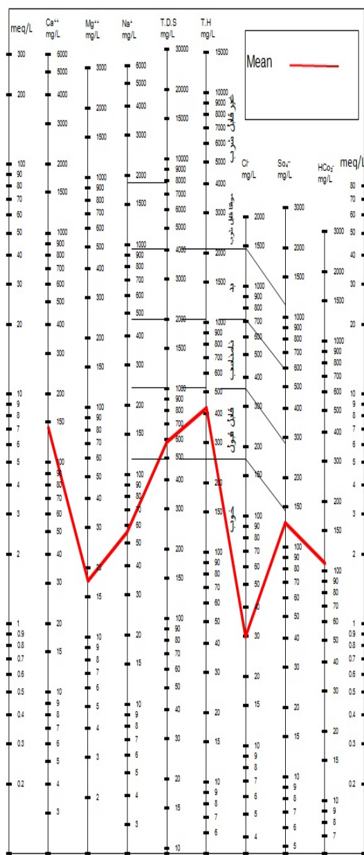
نمودار ۸- دیاگرام شولبرای چاه آب شرب منطقه ی هنزک
