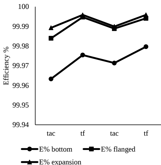
شکل ۴: میانگین راندمان فیلتراسیون در سه حالت ورودی در زمان اندازه‌گیری اول
