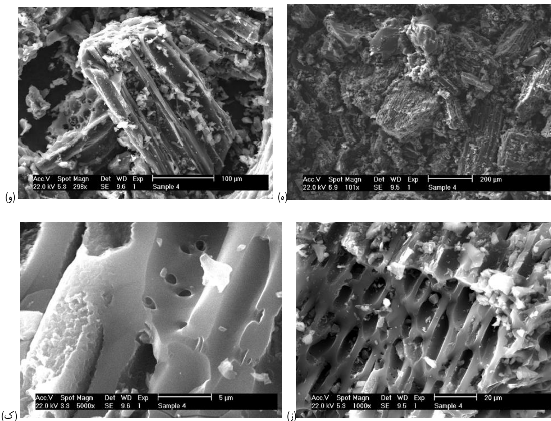
شکل ۴- ادامه- تصاویر SEM کربن فعال‌های ساخته شده از چوب سالم (S) اصلاح نشده (الف-د) و اصلاح شده با پلاسما تحت شرایط ولتاژ ۲ کیلو ولت و زمان ۲۰ دقیقه (ه-ک)
