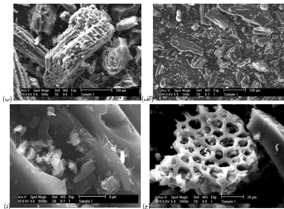
شکل ۴- تصاویر SEM کربن فعال‌های ساخته شده از چوب سالم (S) اصلاح نشده (الف) و اصلاح شده با پلازما تحت شرایط ولتاژ ۲ کیلو ولت و زمان ۲۰ دقیقه (د-ه)
