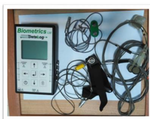
شکل ۳- دستگاه الکترومیوگرافی مدل Data Log Biometrics Ltd مورد استفاده در این مطالعه
