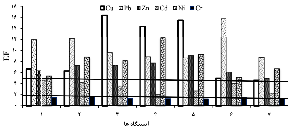
نمودار ۵- نمودار مقادیر EF فلزات مورد مطالعه در ایستگاه‌های مختلف
