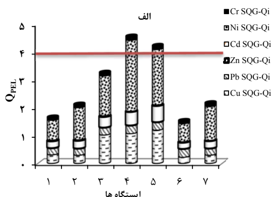
نمودار ۱- (الف) نمودار تجمعی مقادیر Q_{PEL} در هر ایستگاه و (ب) نمودار تجمعی مقادیر Q_{TEL} در هر ایستگاه
