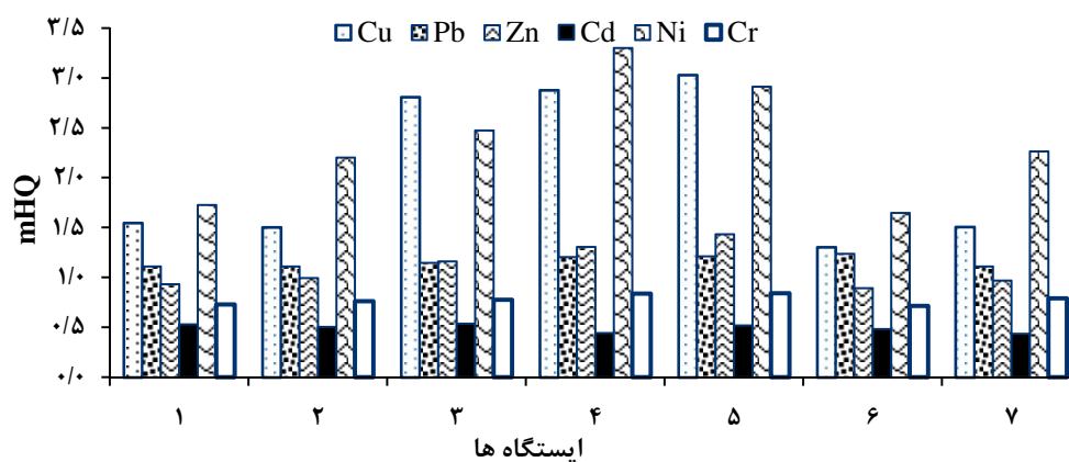
نمودار ۲- نمودار بر خه خطر فلزات مختلف در منطقه مورد مطالعه
