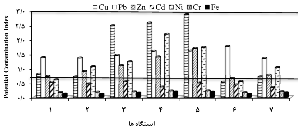
نمودار ۶- نمودار شاخص PCI در ایستگاه‌های مختلف
