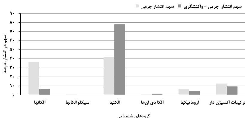
نمودار ۲- سهم گروه‌های شیمیایی در فهرست جرمی - واکنشگری (درصد) و فهرست جرمی (درصد) ترکیبات آلی منتشره در پارس جنوبی
