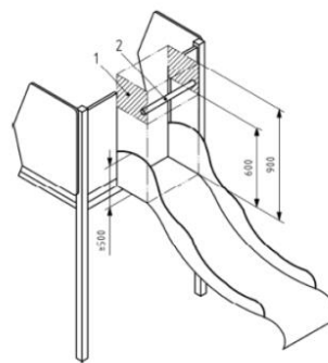
شکل ۱. نمونه ابعاد مربوط به ایمنی سرسره ها
