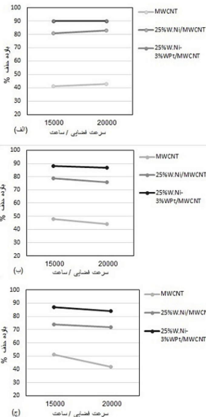
شکل ۷. بازده حذف کاتالیستی در سرعت های فضایی ۱۵۰۰۰-۲۰۰۰۰ hr/m³، دمای ۲۵۰°C و غلظت های (الف) ۳۰۰۰ ppm (ب) ۴۰۰۰ ppm (ج) ۵۰۰۰ ppm.
