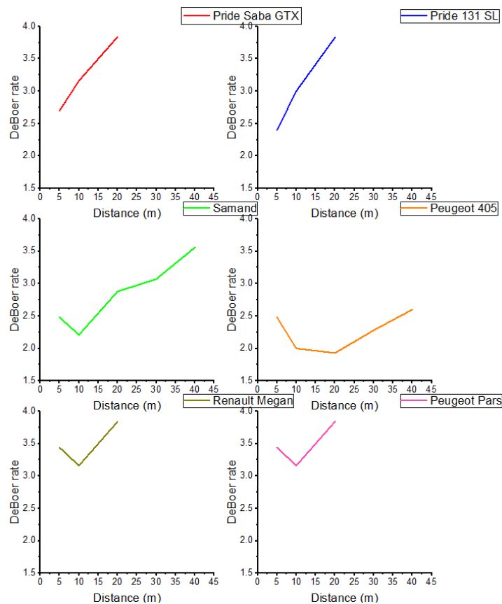
شکل ۴: سطح خیرگی آزاردهنده خودروهای بررسی شده در حالت نورپایین در درخشندگی زمینه ۱ کاندا بر مترمربع
