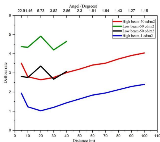
شکل ۶: میانگین خیرگی آزردهنده چراغ خودروها در زوایا و فواصل مختلف اندازه‌گیری در حالت نورپایین و نوربالا
