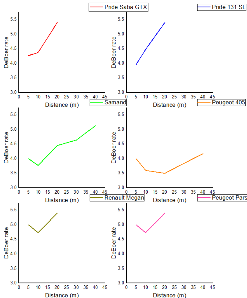
شکل ۵: سطح خیرگی آزردهنده خودروهای بررسی شده در حالت نورپایین در درخشندگی زمینه ۵۰ کاندلا بر مترمربع
