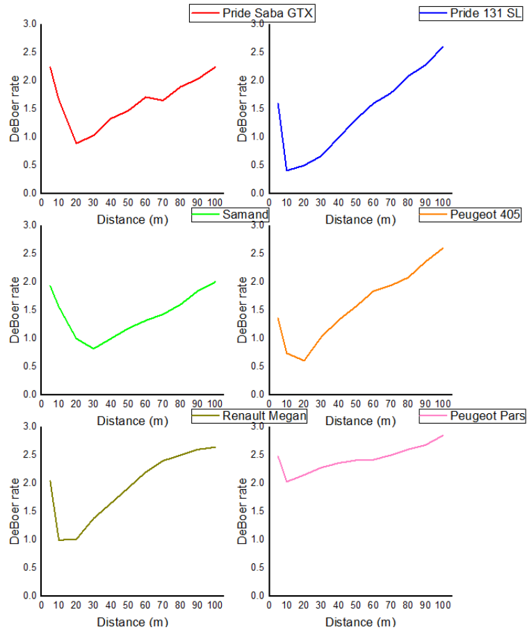
شکل ۳: سطح خیرگی آزاردهنده خودروهای بررسی شده در حالت نوربالا در درخشندگی زمینه ۱ کاندا بر مترمربع
