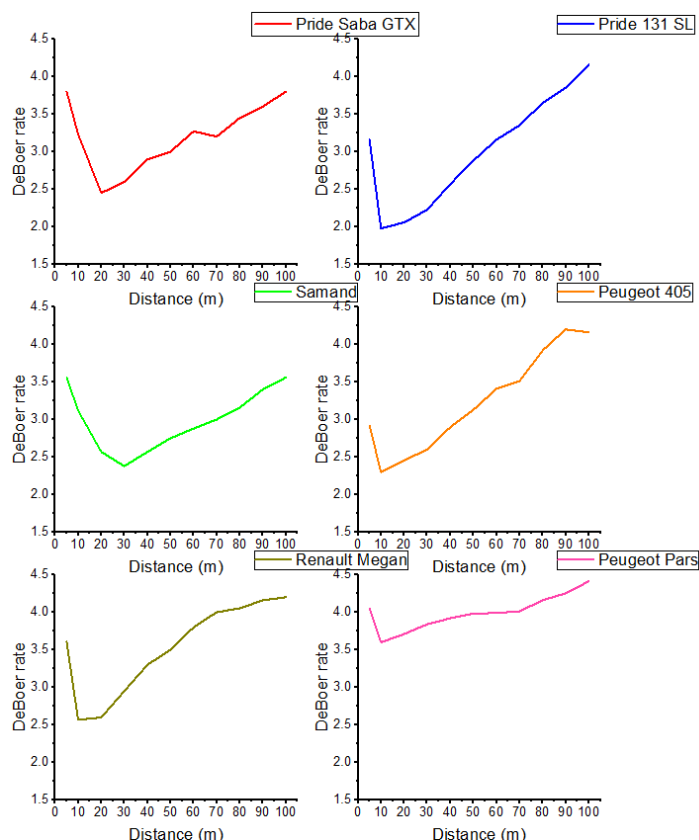
شکل ۲: سطح خیرگی آزاددهنده خودروهای بررسی‌شده در حالت نوربالا در درخشندگی زمینه ۵۰ کاندلا بر مترمربع
