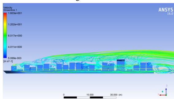
شکل ۱۲- تصویر خطوط جریان از روی شناور
