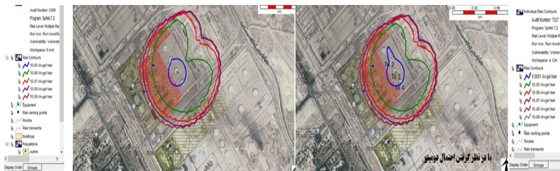
تصویر ۴. تراز ریسک فردی ناشی مخزن TK3 با و بدون در نظر گرفتن اثرات دومینو
