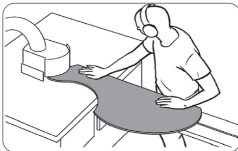
۳۳-۳. استفاده از محافظ حلقوی در فرزکاری
