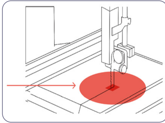
۳-۹. محدوده خطر در اره نواری
