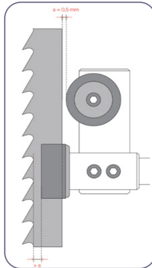
۳-۱۰. جایگاه نوردهای هدایت کننده در اره نواری
