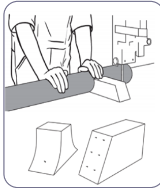
۳-۱۵. برش عرضی قطعات استوانه‌ای شکل
