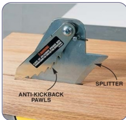
شکل ۴-۶. جداکننده و چنگک ضد برگشت
