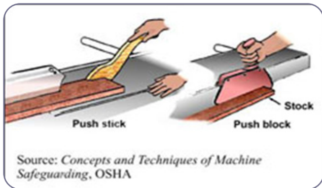
شکل ۲-۴. چوب یا بلوک فشارآور (راهنما)
