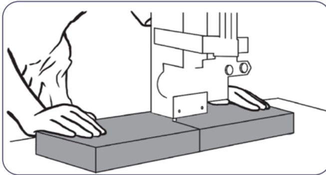
۳-۱۳. طرز قرار گرفتن دست‌ها در برش عرضی
