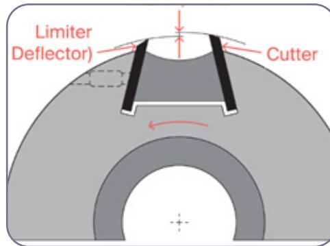
۳-۲۷. اختلاف ارتفاع لبه محدودکننده با تیغه
