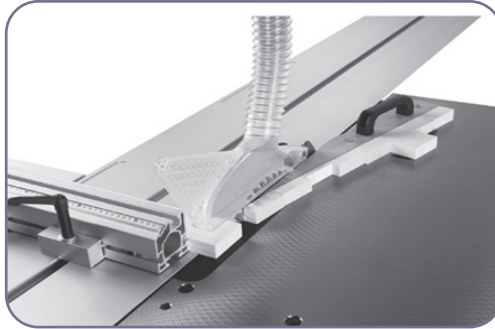
۳-۷. استفاده از گوه جداکننده در برش عرضی
