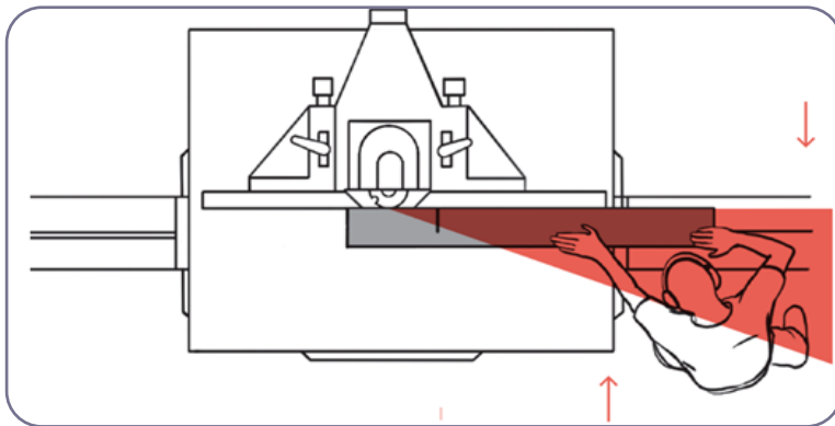
۲۵-۳. محدوده خطر در دستگاه فرز میزی
