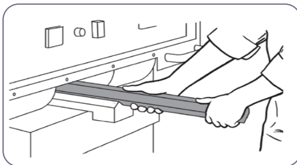
۳-۳۶. استفاده از تکیه‌گاه ثابت در دستگاه گندگی
