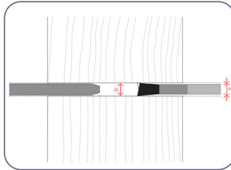
۲-۳. طرح شماتیک تیغه و چاقویی در چوب
