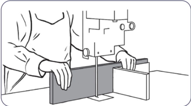
۳-۱۴. استفاده از بلوک چوبی در برش عرضی عمودی
