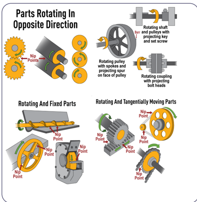
شکل ۴-۴. نقاط فشار یا پینچ. برگرفته از (OSHAcademy (Geigle Safety Group)
